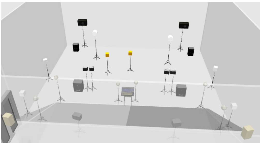
plan de l'acousmonium à l'Audible Festival
